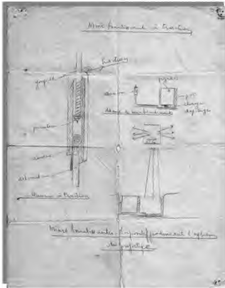
مخطط لطريقة تفجير لغم مرتد (قافز). أرشيف شخصي خاص بالمجاهد بلحسن بالي
